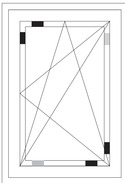
Cercevea oscilo-batantă
