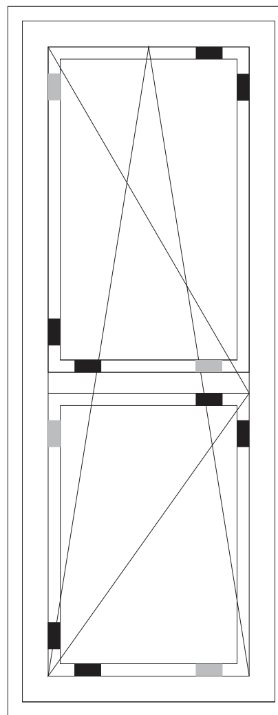
Cercevea batantă
